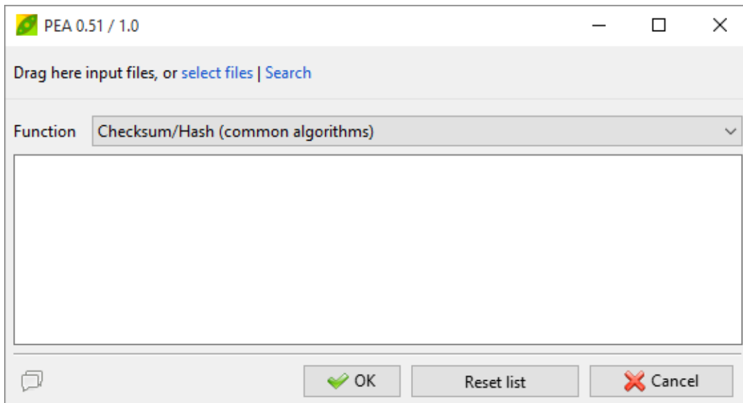
Image 21: PeaUtils
