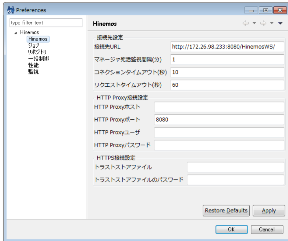
図 9-3 Hinemosマネージャ死活監視間隔
